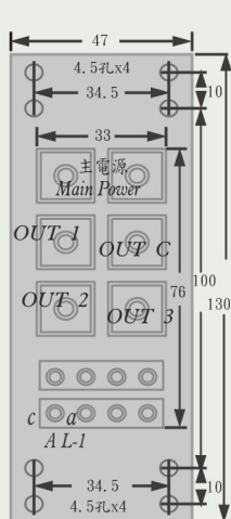
單組出線說明 Cable Connection
