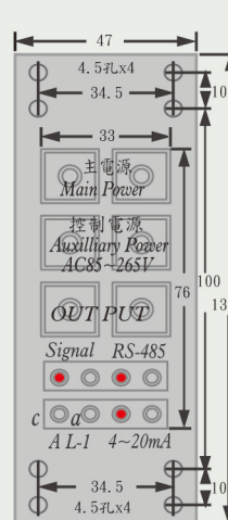
單組出線說明 Cable Connection
