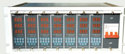
6點控制箱 6 Zones Control Box
